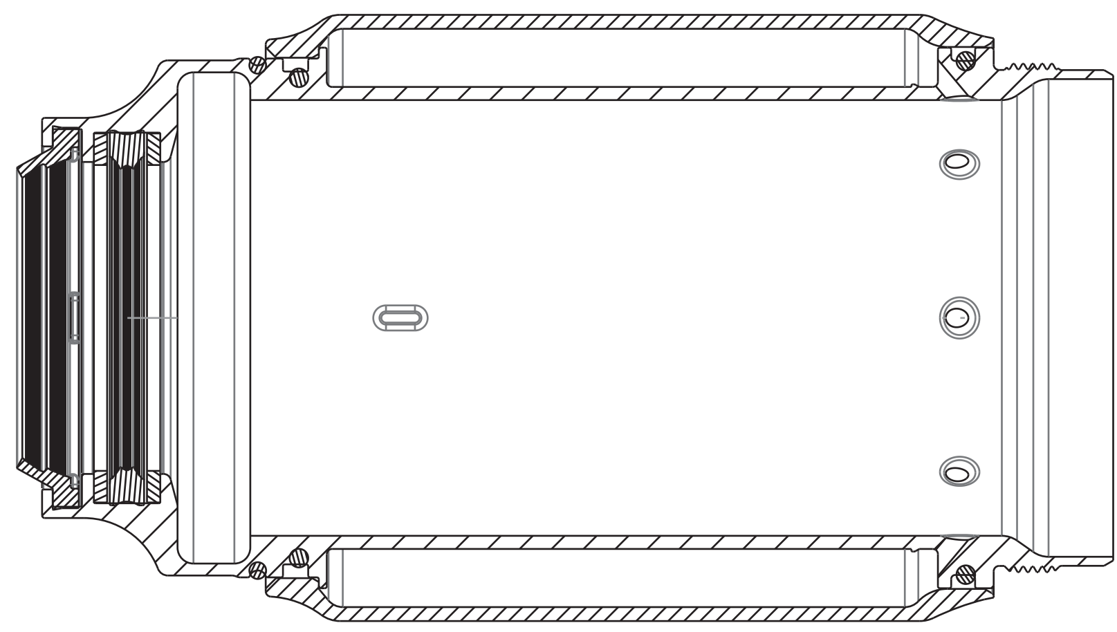
SECTION A-A
